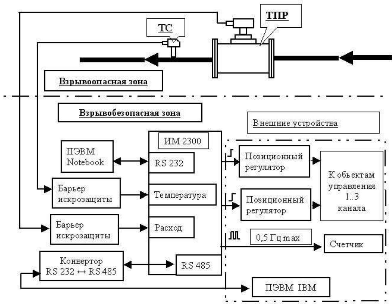
Схема взаимодействия расходомера с внешними устройствами.
