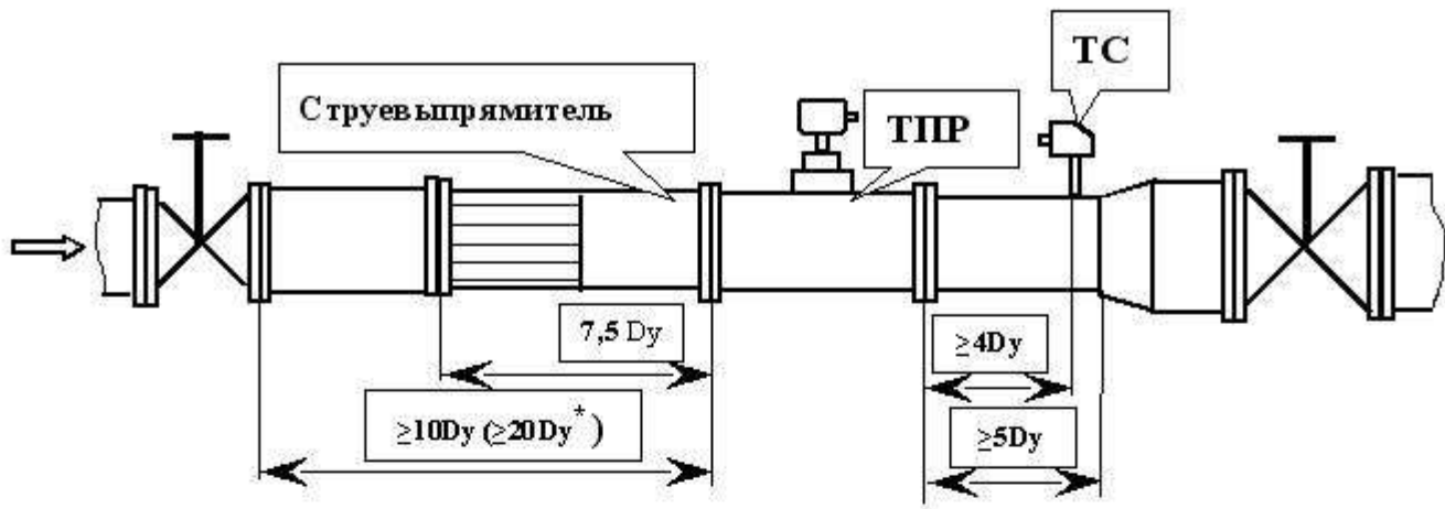
Монтаж ТПР на трубопроводе .
